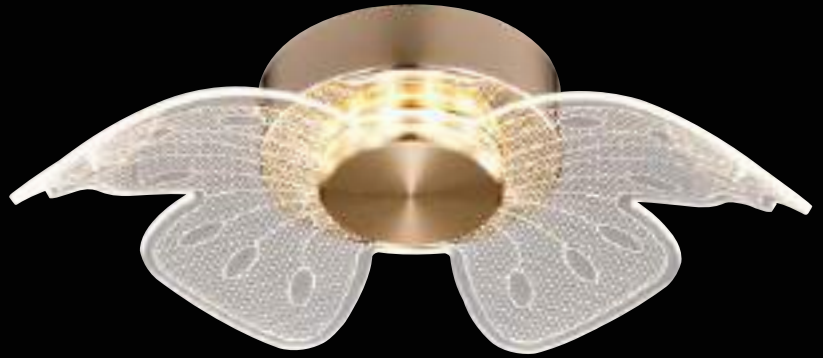
■ PY6-2151 4333 L240 W150 H90mm LED 7W / 三色變光 金屬電鍍 壓克力
