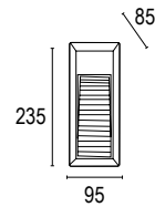
預埋盒尺寸： W85 H225 D86
