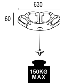
FL-7001-3 107000 Ø630 H60 mm 載重 150 公斤 配置 6 米鋼線 載重物：50~150 公斤
