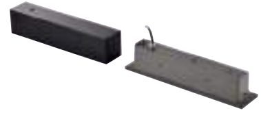
預埋盒尺寸: W312 H61 D68
