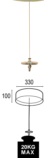
FL-7001-1 53000 Ø330 H100 mm 載重 20 公斤 配置 20 米鋼線 載重物：6~20 公斤
