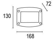
預埋盒尺寸: W160 H96 D75
