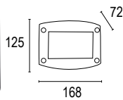
預埋盒尺寸: W160 H96 D75
