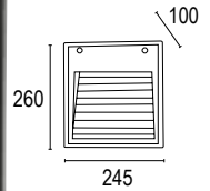
預埋盒尺寸: W220 H240 D110
