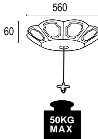
FL-7001-2 62000 Ø560 H60 mm 載重 50 公斤 配置 4 米鋼線 載重物：15~50 公斤
